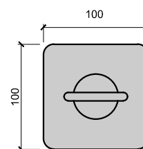
POHLED SHORA
